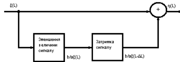
Рис. 3. Структурна схема перетворення сигналу зображення при двоїнь растрових точок
