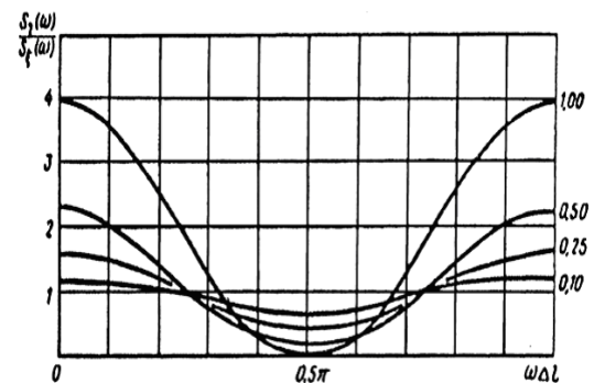
Рис. 4. Відносні зміни енергетичного спектра сигналу зображення при явищі двоєння растрових точок (при \frac{b}{a} = 1,00; 0,50; 0,25; 0,10 )
