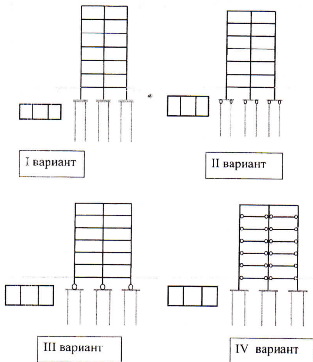
Рис.3 – Возможные варианты расчетных схем проектируемого объекта
