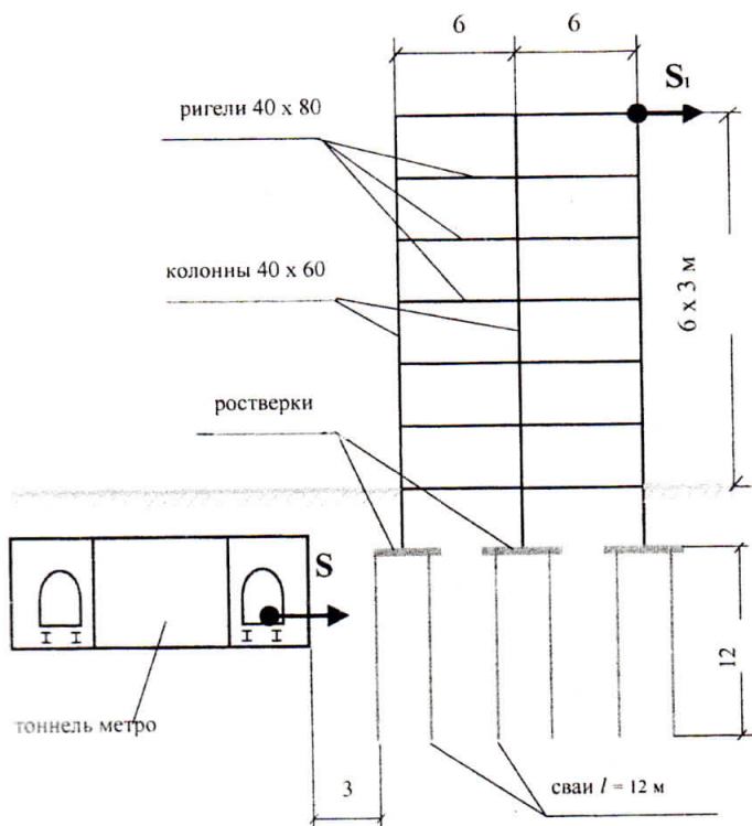
Рис 2 – Расчетная схема объекта проектирования
