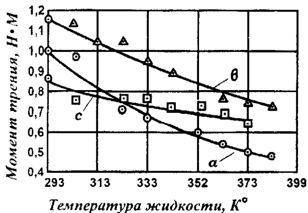
Рис. 1. Изменение момента трения образцов от температуры при трении в жидкости АМГ-10.
