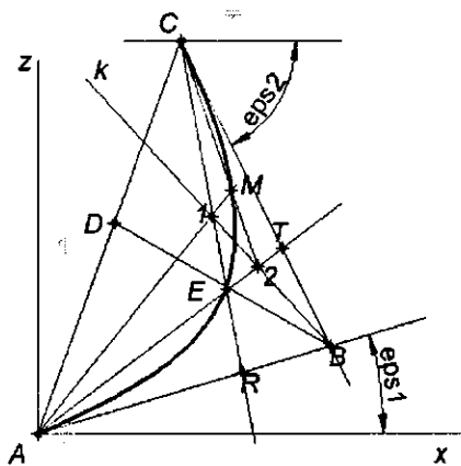
Рис. 2. Проектування напрямних кривих
