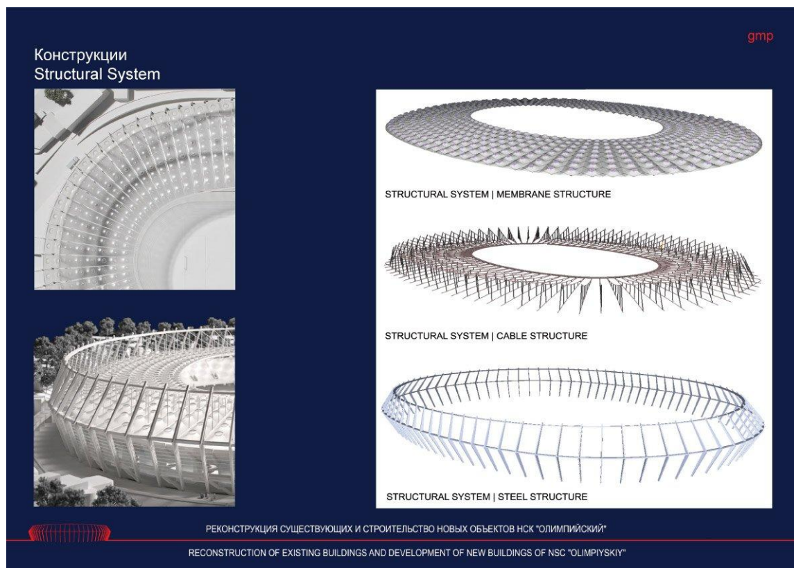
Рис.3. Конструкція даху НСК
