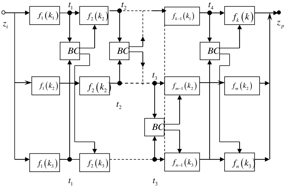
Рис. 1. Блок-схема каналів, що приймають участь у реалізації послуги Z_i в системі зв'язку
