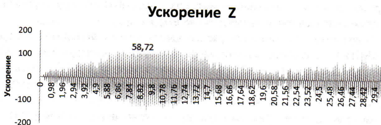
Рис. 2. б - ускорение вдоль оси Z в точке А
