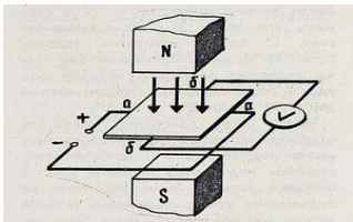
Структура датчика Холла
