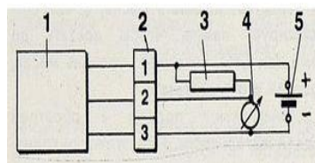
Елементи датчика Холла
