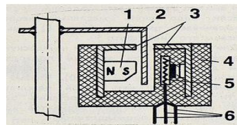
Пристрій датчика Холла
