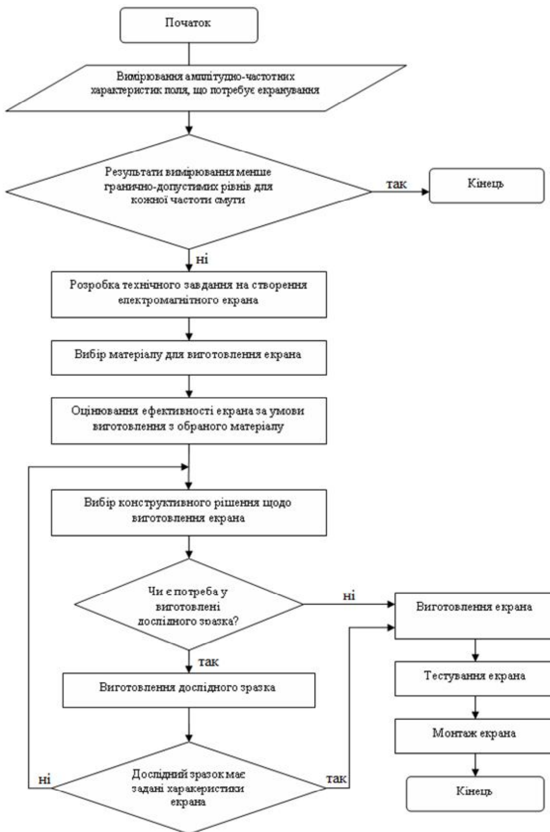
Рис. 3. Схема реалізації електромагнітного екранування потрібної ефективності
