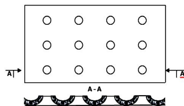
Рис. 3. Фронтальний вигляд та розріз поглинального електромагнітного екрана
