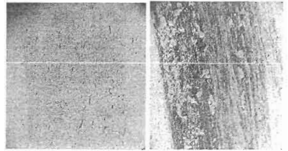
Рис. 4. Топографія поверхні тертя на склі сталлю 3: а) з напрямом магнітного поля N->S т. № 1, б) при напрямі S->N магнітного поля в т. № 3.
