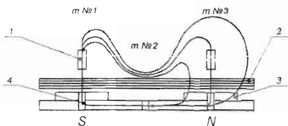
Рис. 1. Схема проходження магнітних силових ліній через стальний зразок: 1 – зразок, 2 – скло, 3 – магніт, 4 – отвір.
