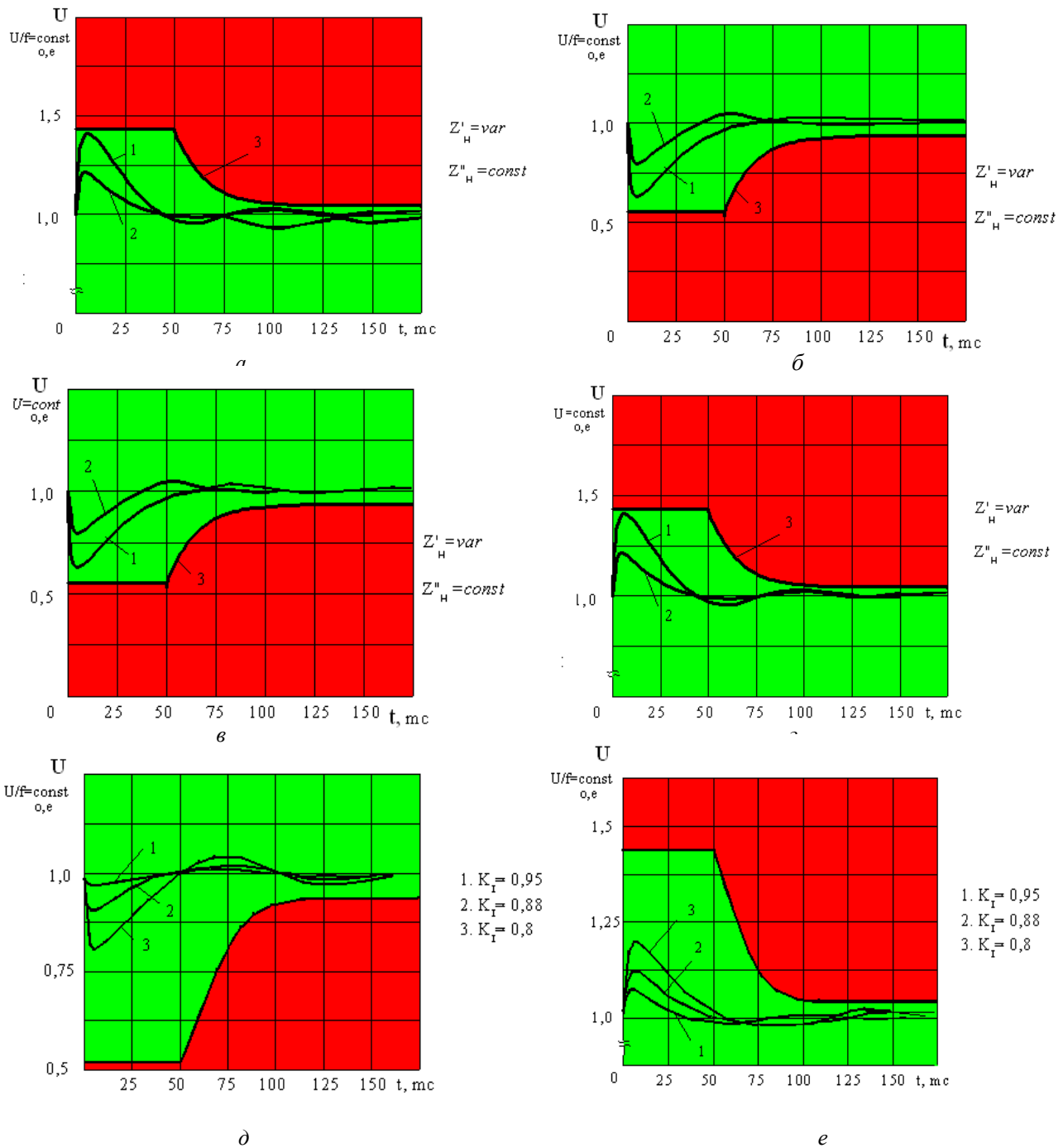
Рис. 4. Перехідні процеси в каналах СГ за різних режимах роботи:
