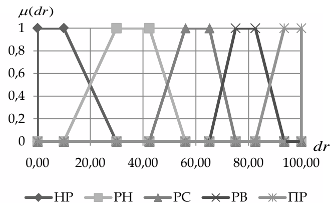
Рис. 2. Термы эталонных значений неравномерно распределенных НЧ для ЛП DR при \underline{T}_{DR}^{(4)} и \underline{T}_{DR}^{(5)}
