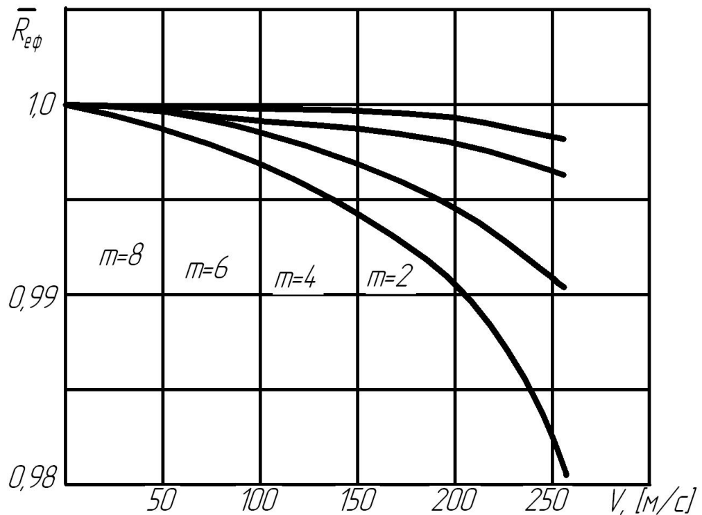
Рис.1.13. Вплив зовнішнього опору мотогондоли на ефективну тягу двоконтурного двигуна (подовження мотогондоли \lambda=8 )
