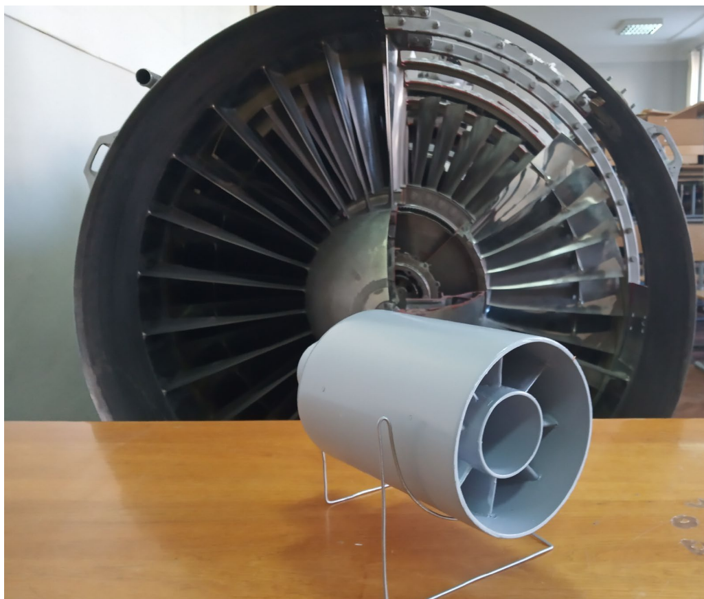
Рис.3.10. Модель мотогондoli ТРДД с традиційним переднім розташуванням вентилятора
