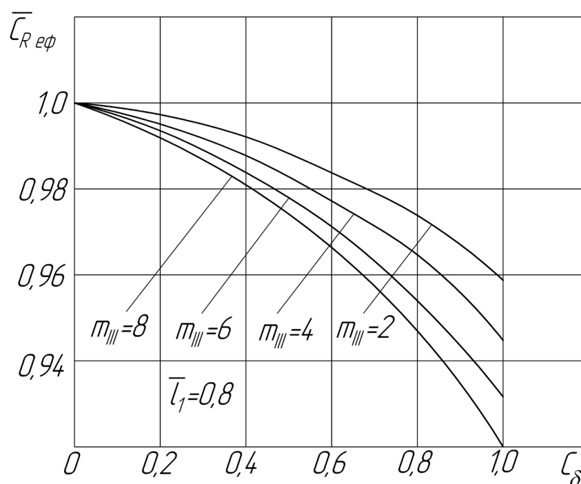
Рис.6.12. Вплив управління примежовим шаром на поверхні мотогондולי газогенератора силової установки з турбовентиляторною приставкою на ефективну питому витрату палива триконтурного двигуна (подовження мотогондולי \lambda=8 )
