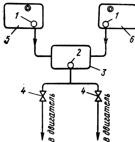
Рис. 1.1. Схема подачі пального з одним витратним баком
