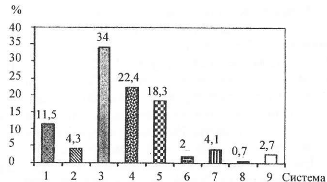
Рис. 4.1. Розподіл інцидентів за системами ПС через провину ІАС: 1 — масляна система; 2 — паливна система; 3 — система шасі; 4 — планерувальна система; 5 — двигун та його агрегати; 6 — гідросистема; 7 — система реверсу; 8 — протиобліднювальна система; 9 — автоматична бортова система керування
