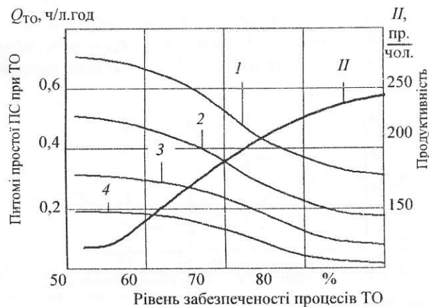
Рис 4.15. Залежність простоїв ПС під час ТО й продуктивність праці від рівня забезпеченості процесів ТО: 1 — дальньомагістральний літак; 2 — середньомагістральний літак; 3 — ближньомагістральний літак; 4 — літак місцевих повітряних ліній
