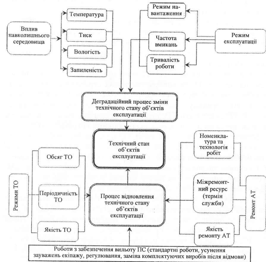
Рис. 1.2. Процес зміни технічного стану функціональних систем ПС
