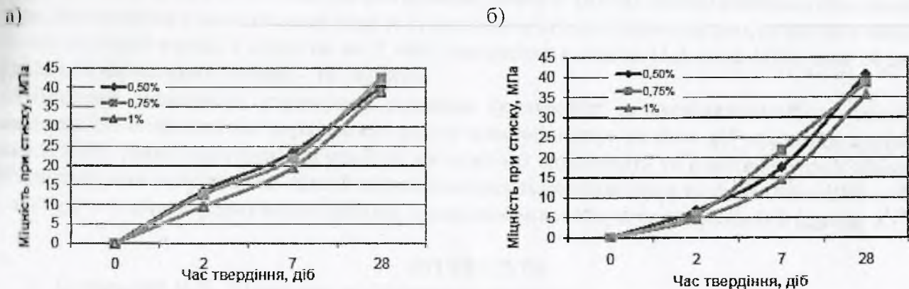
Рисунок 5 Залежність зміни міцності цементного каменю у часі від вмісту і величини \text{pH} пластифікатора в складі лужного золівмісного цементу: а \text{pH} = 8,25 , б \text{pH} = 9,9
