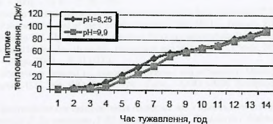
Рисунок 6 Питоме тепловиділення в системі «зола портландцементний клинкер лужний компонент добавка ПАР» залежно від величини рН пластифікатора
