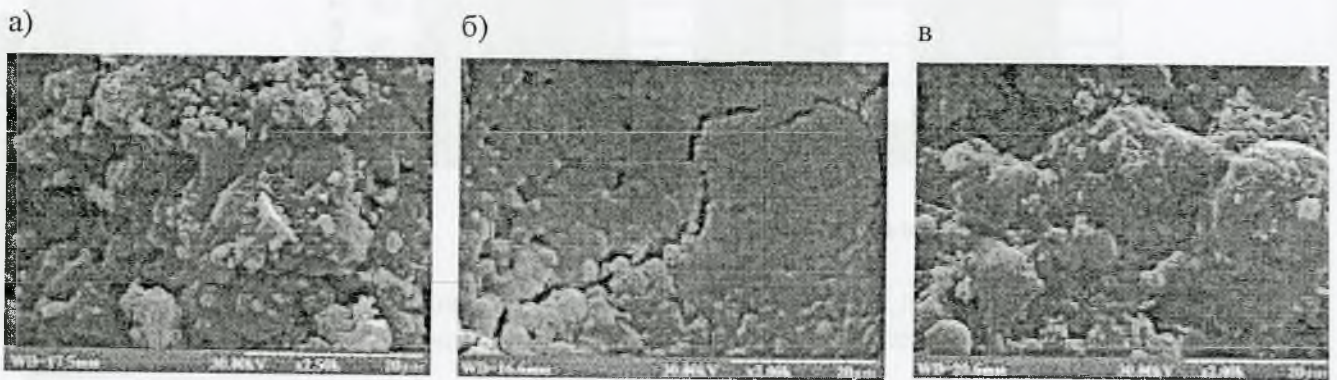
Рисунок 2 Фотографії поверхні сколу штучного каменю на основі цементів, що містять лужний компонент, після 28-ми діб тверднення: а \text{Na}_2\text{CO}_3 5 % за масою; б \text{Na}_2\text{SiO}_3 \cdot 5\text{H}_2\text{O} 8 % за масою; в \text{Na}_2\text{CO}_3 (4 % + \text{Na}_2\text{SiO}_3 \cdot 5\text{H}_2\text{O} 6 %).
