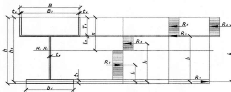
Рис. 1 - Схема внутрішніх зусиль у нормальному перерізі Умови статички (7):
